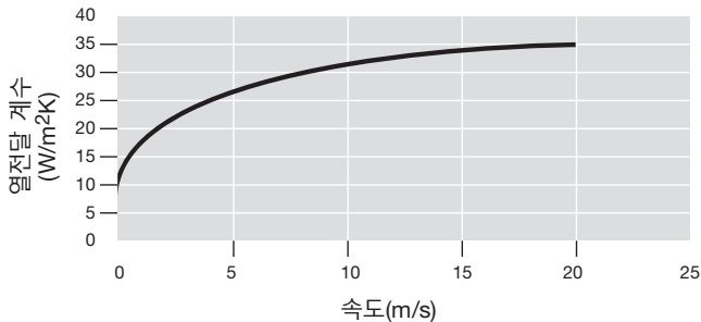
공기-열전달 계수 근사치
