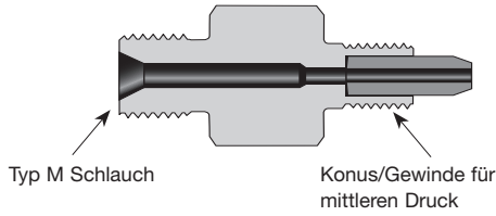
Typ M Schlauch auf Konus/Gewinderohr für mittleren Druck
