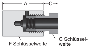
Mitteldruck-Konfiguration abgebildet
