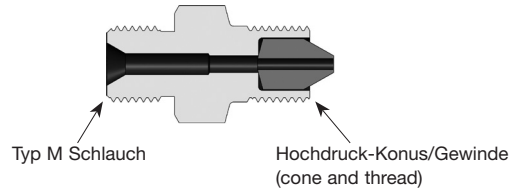
Typ M Schlauch auf Konus/Gewinderohr für hohen Druck
