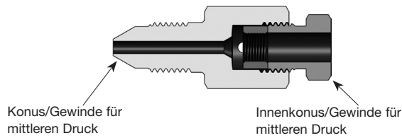
Die Abbildung zeigt einen einteiligen Außengewindekonus Siehe Zusatz -S1 für weitere Informationen.
