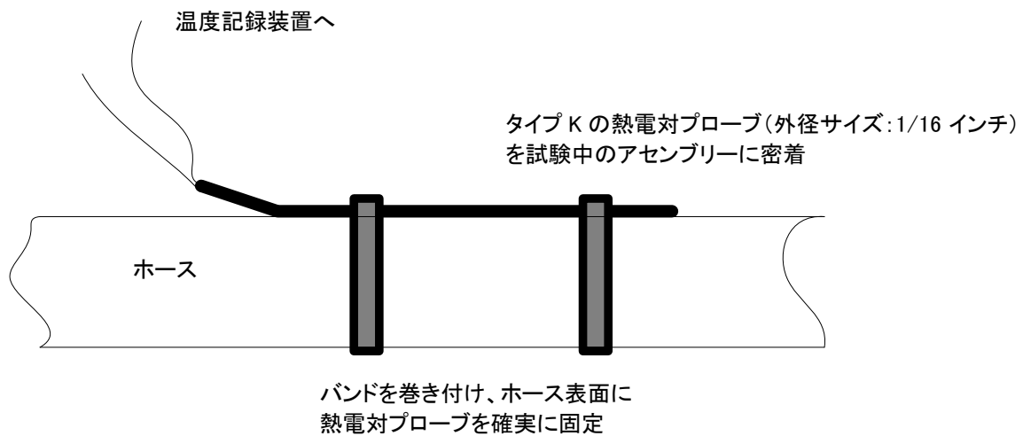
図 2: 熱電対のホース表面への取り付け図
