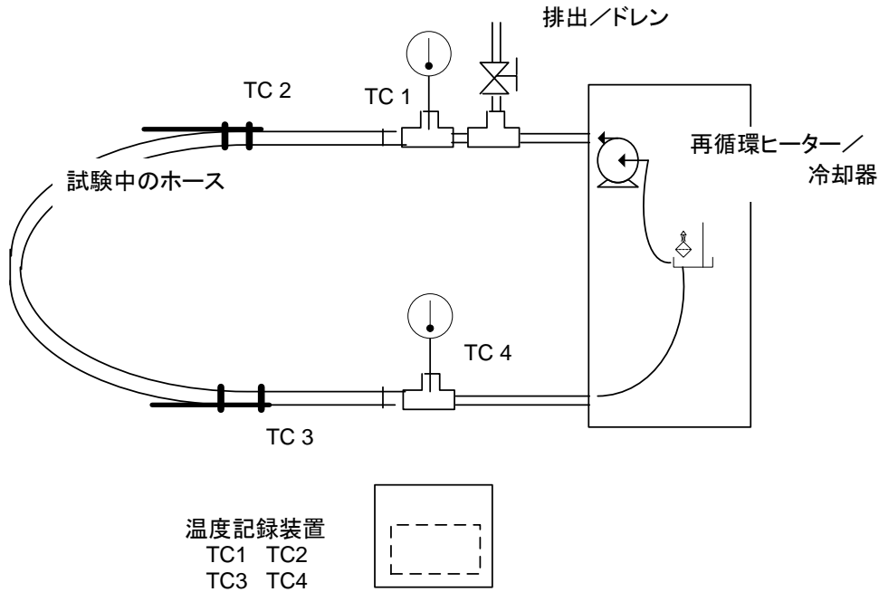
図 1: 試験流路図
